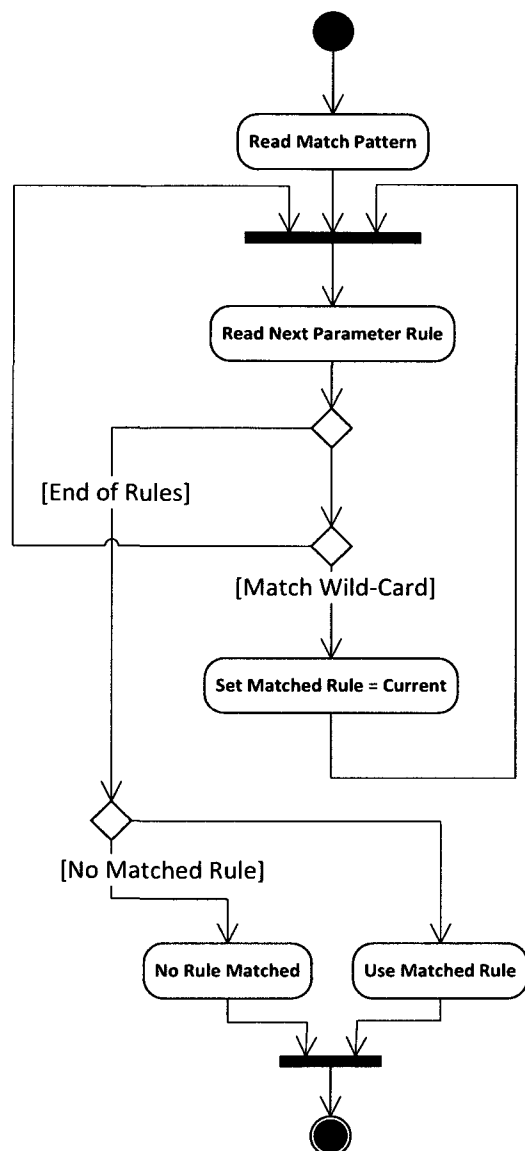
Figure 29. Parameter mask matching algorithm.
